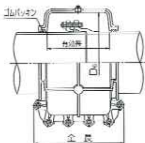
呼び径350～700
