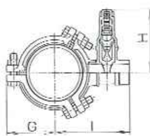
SUN型
