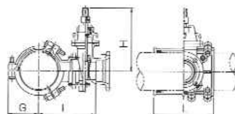
ヤノT字管VK型
