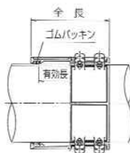
呼び径50～350
