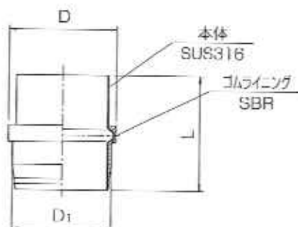
呼び径40・50
