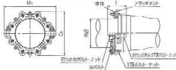
呼び径300～450
