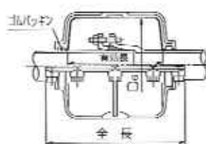
呼び径75～300
