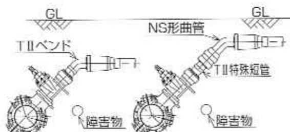
TⅡベンド使用時
