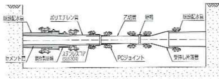
■パイプリバー工事立坑内標準配管図
