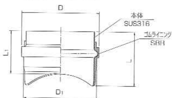
呼び径75・100・150
