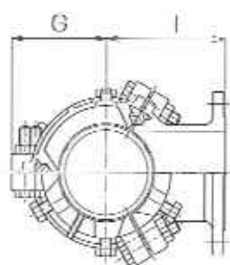
同口径ヤノT字管F型
