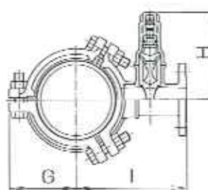
SF型
