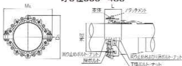
呼び径300~450
