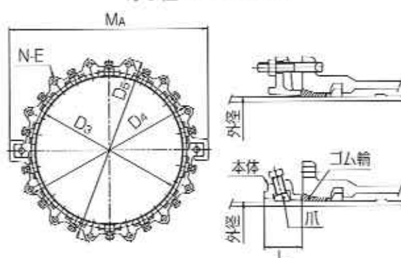
呼び径500～1000
