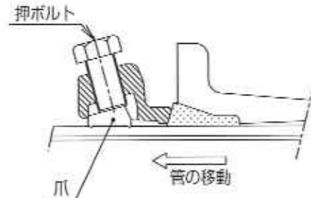
水圧負荷時
