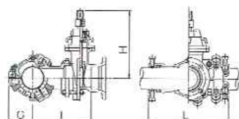
同口径ヤノT字管VK型
